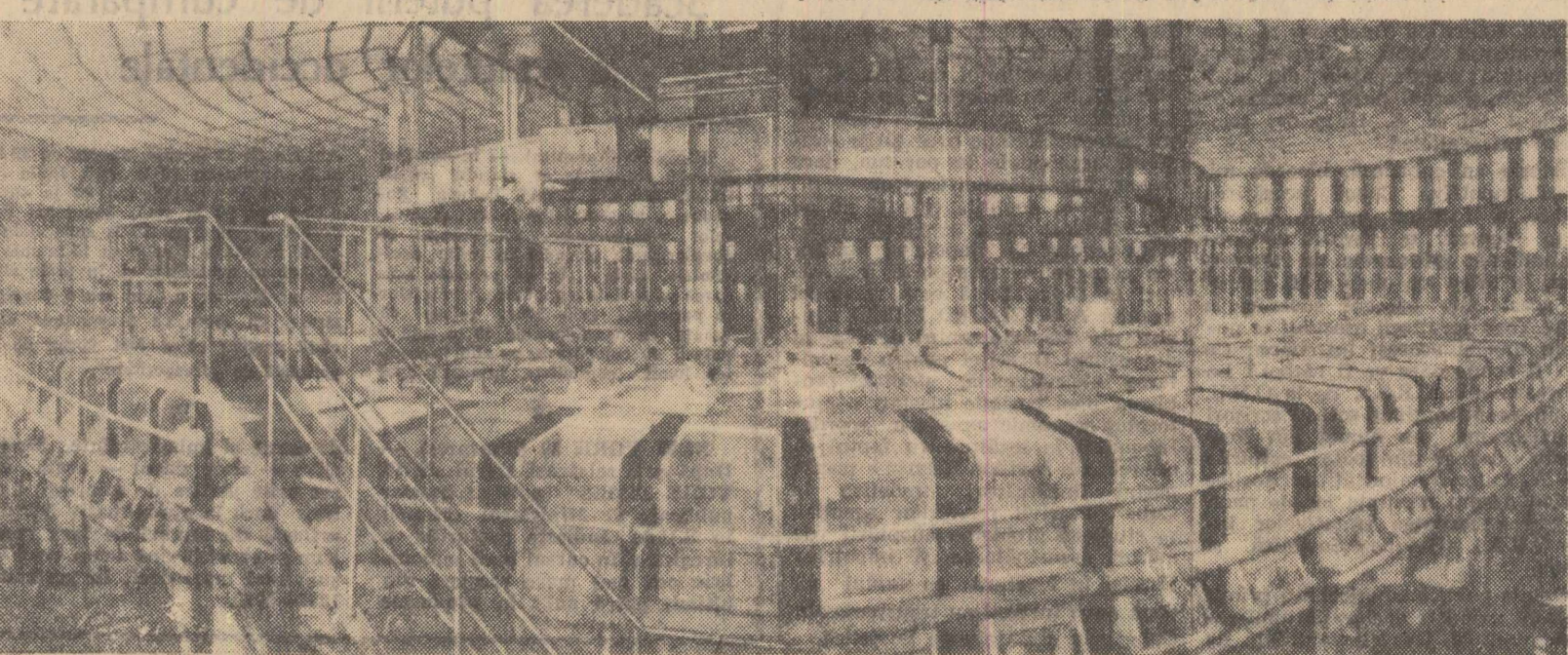
Aspect general al magnetului circular — în greutate de 36.000 tone — al sincrozotronului de la Dubna
