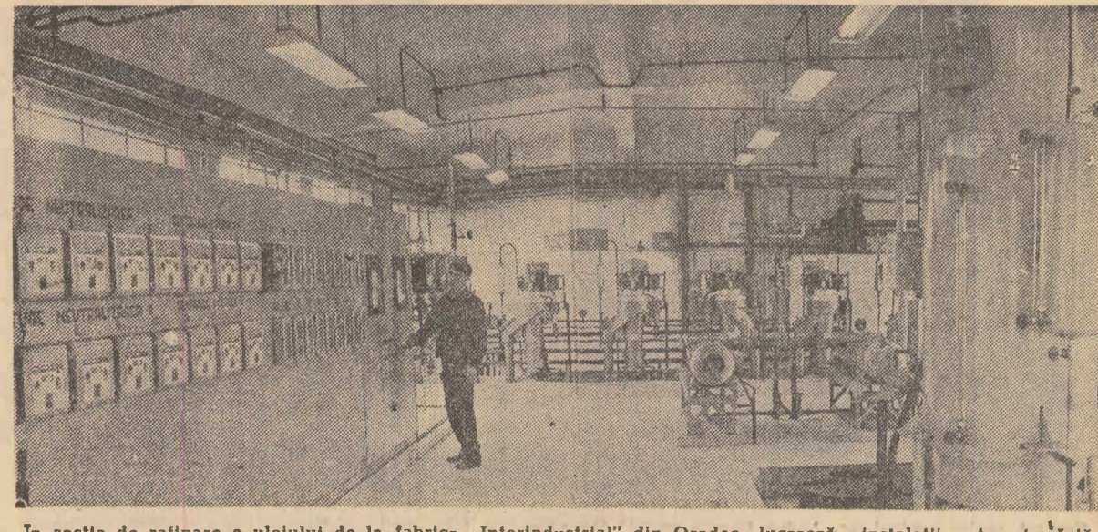
În secția de rafinare a uleiului de la fabrica „Interindustrial” din Oradea, lucrează instalații automate. Tatăl tânărului Nicolae Igna, ajutor centrifug, supraveghează instalațiile
