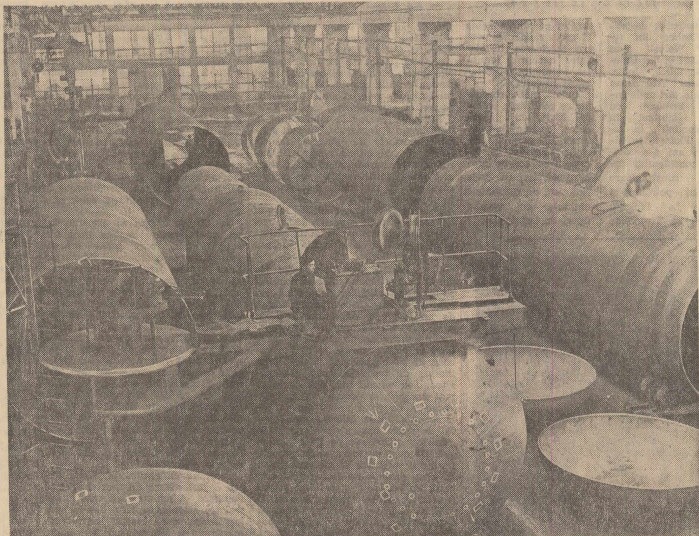
Ca rezultat al promovării procedeele tehnologice moderne, la uzinele „Vulcan” din București, în secția cazangerie, a fost organizată după principii moderne, o linie tehnologică de sudură automată. Iată un aspect al acestei linii de producție. La agregatul de sudură lucrează tinerii C. Paul și Vasile Tăbăraș.
