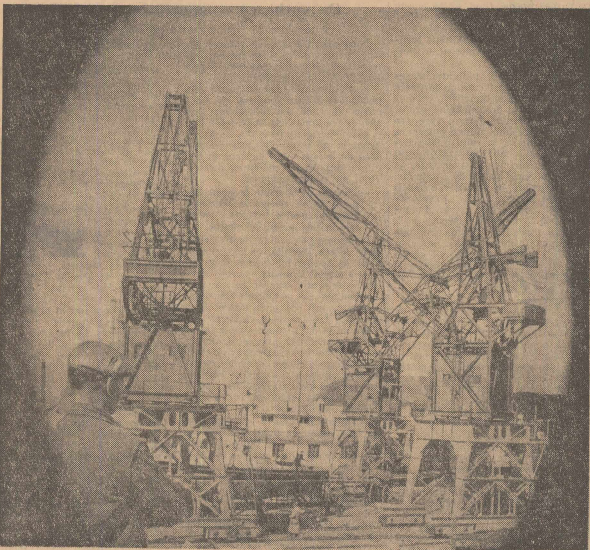
Vedere parțială a șantierului naval Oltenița
