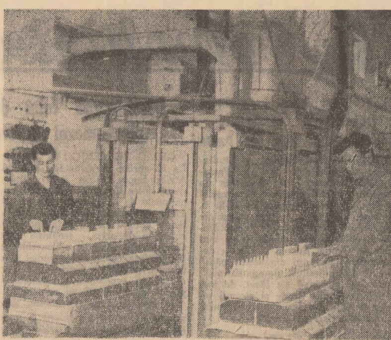
La cuptorul-tunel pentru arderea izolatoarelor de la fabrica de buji și piese auto „Triumf” din Cluj, controlorul de calitate Georgehe Maris împreună cu muncitorul Ion Cudor, fac ultimul control al izolatoarelor înainte de introducerea în cuptor
