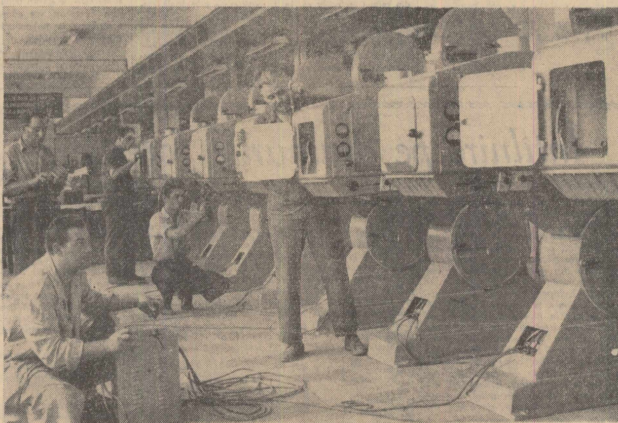
Recent, la întreprinderea „Industria optică română” din Capitală, a intrat în fabricația de serie aparatul perfecționat de protecție cinematografică T. 6. Aparatul se pretează la protecții pe ecran normal, pe ecran lat și cinematograf și cu sunet stereofonic, fiind destinat celor mai moderne săli de cinematograf atît de la oraș cît și de la sat. În cliseu: echipa de montori condusă de Aurel Arghireanu finisînd un lot de aparate T. 6.
