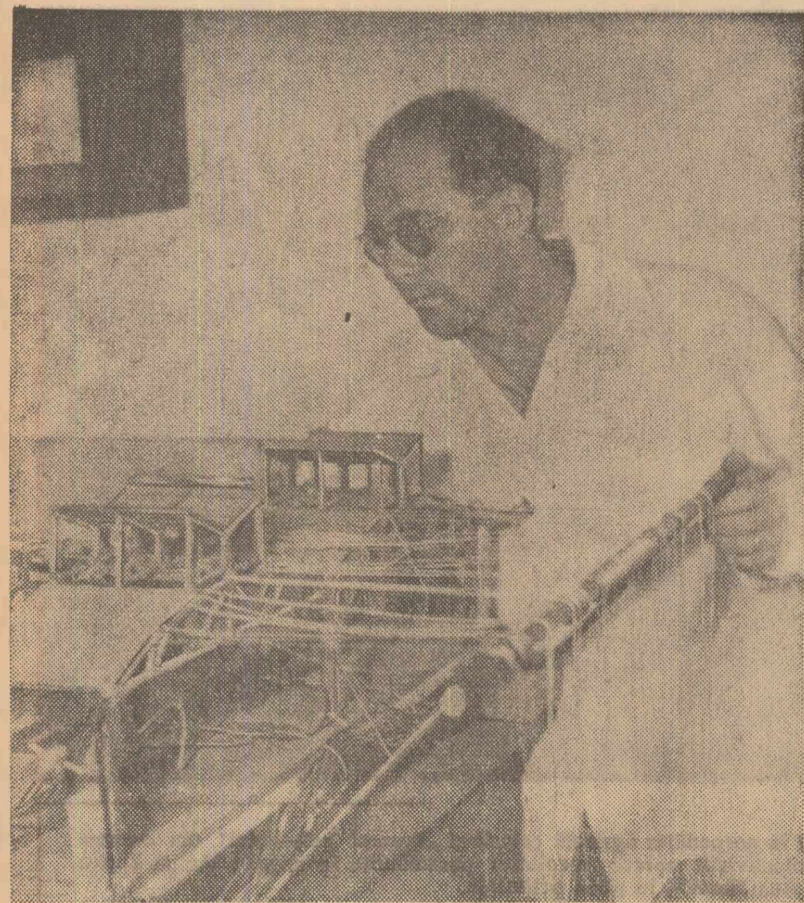
Instantaneu la Institutul de cercetări în construcții și economia construcțiilor — INCERC — : În laborator de studii pe modele, ing. Eduard Nicolau, efectuează măsurători la o hală industrială tip, pentru a-și stabili capacitatea de rezistență.
