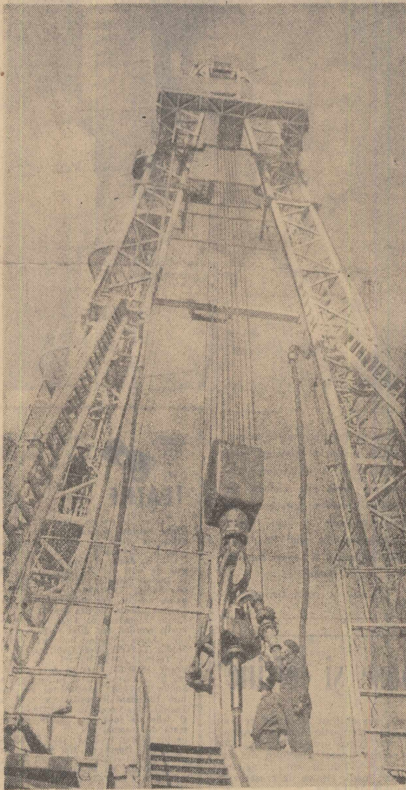
Se forează cu o instalație de tip 3 DH, instalație cu înalte calități tehnice, realizată la uzinele constructoare de utilaj petrolifer „I. Măi”. Ploiești. În prim plan sondei din brigada condusă de Gh. Dumitru, în timpul procesului de forare.
