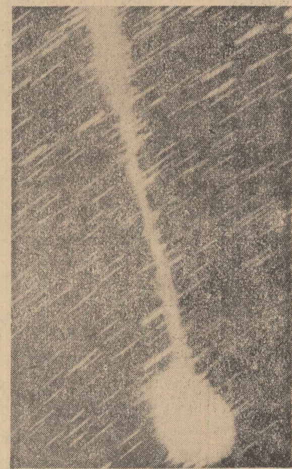
Fotografia alăturată publicată săptămîna aceasta în S.U.A., înfățișează cometa „Burnham 1960 II”, a cărei „coadă” are remarcabilă lungime de 18 milioane de mile. Imaginea acestei comete reprezintă un interes deosebit pentru astronomie.
