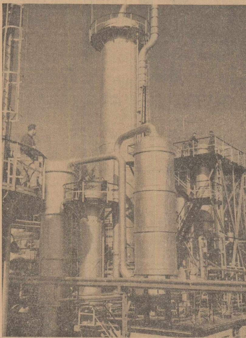
Recent la Combinatul chimic Victoria a intrat în funcțiune o instalație de formol. În cișeu: Un aspect al acestei instalații.
