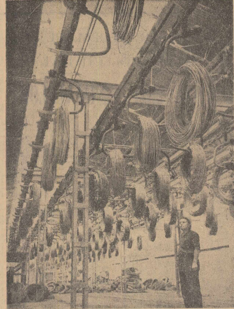
La „Industria sirnei” din Cimpia Turzii funcționează un transportor al colacilor de sirni. Această mecanizare face posibilă răcirea uniformă a firului de sirni pe toată lungimea sa, îmbunătățind totodată condițiile de lucru. În clișeu: Vedere a transportorului.
