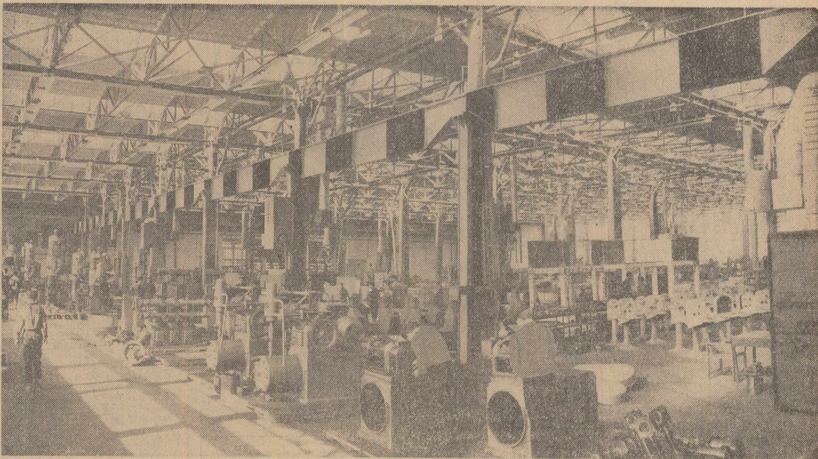
La uzinele „Tehnofrig” din Cluj a fost recent dată în folosință o nouă și modernă hală de fabricație. În clișeu: Aspect din hală unde se produc compresoare frigorifice.
