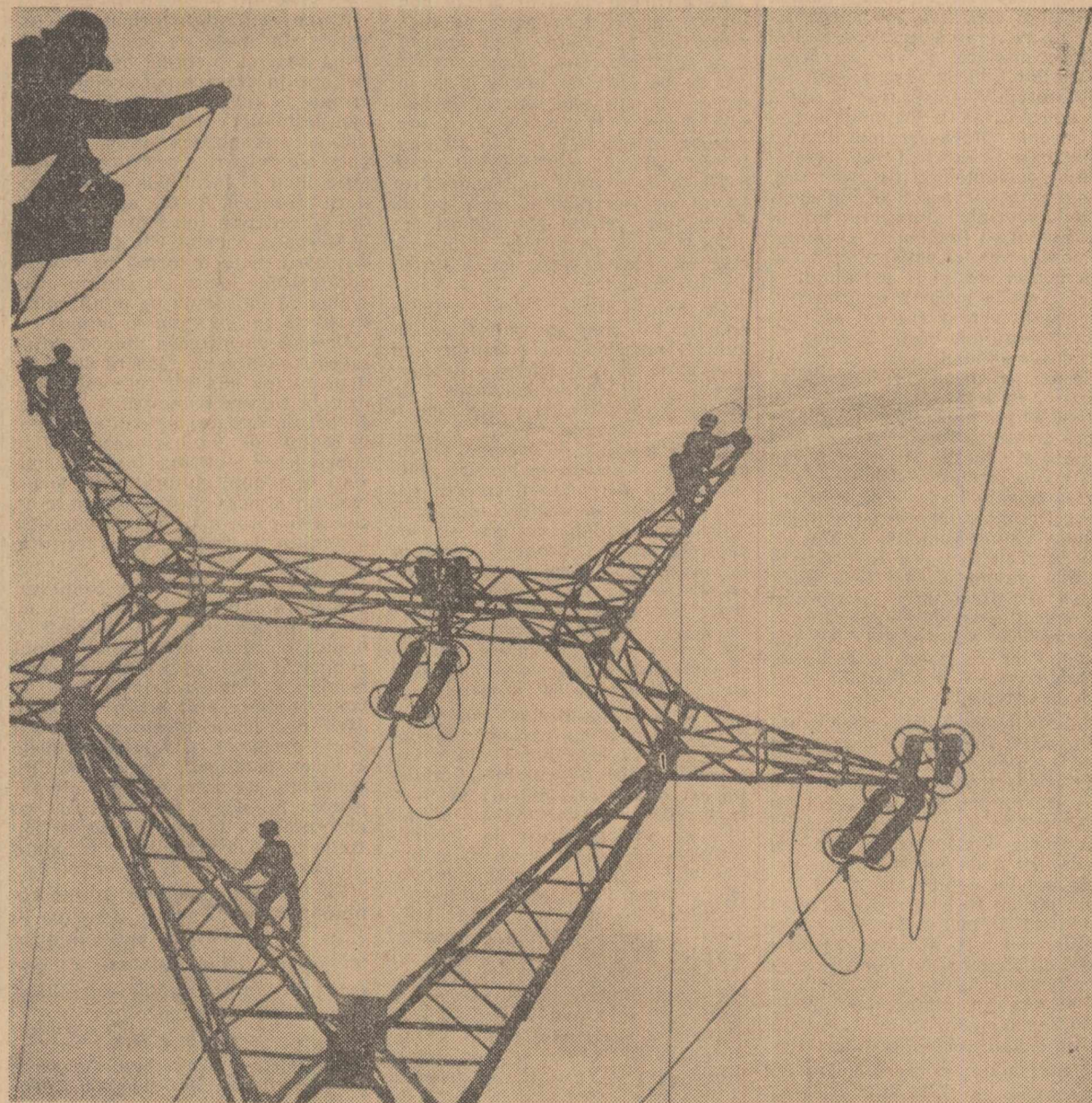
Oameni la înălțimi. Linieri' lucrînd la montarea unei linii de înaltă tensiune
