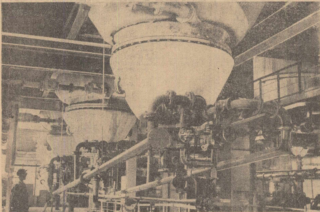
Uzinele de produse sodice Govora. Aspect din secția de fabricare a sodei caustice
