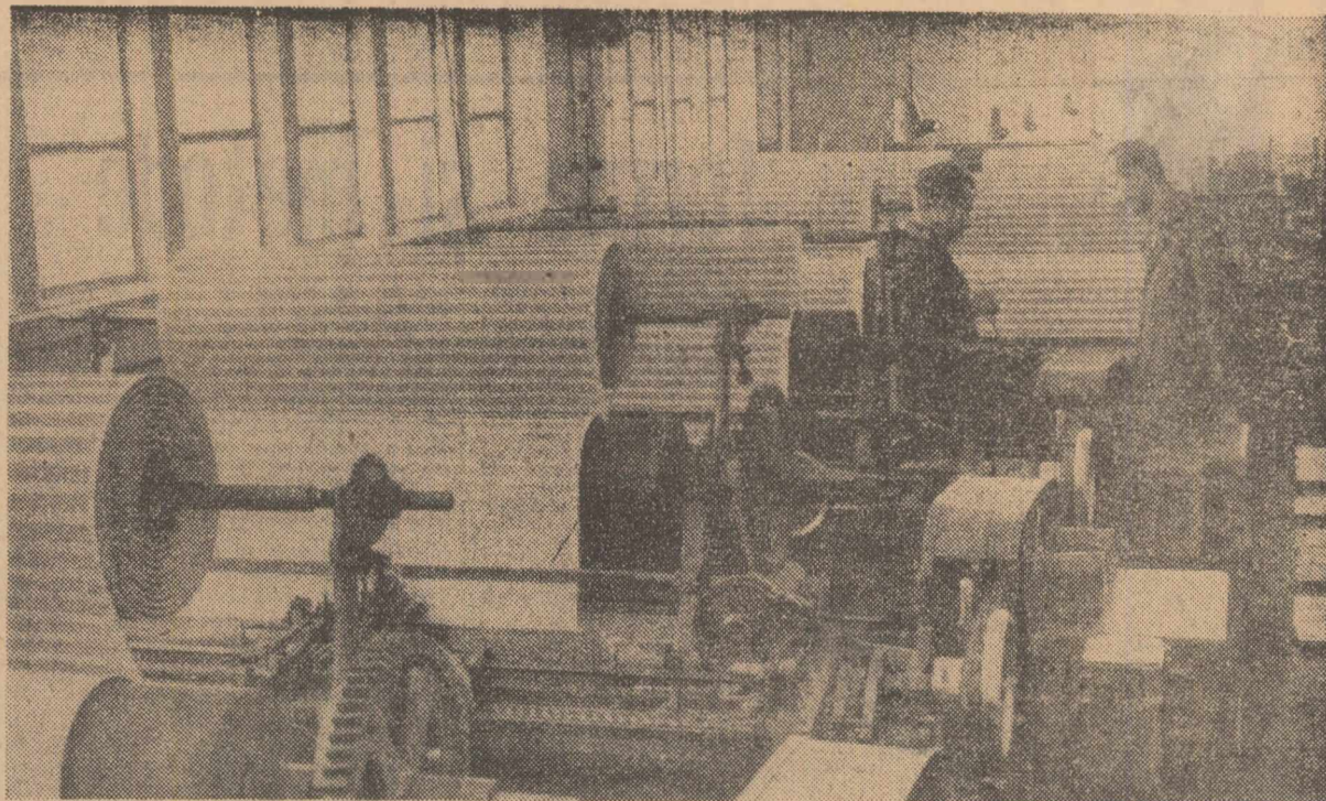
La Fabrica „Metalotehnică” din Tg. Mureș se produc piese de schimb și utilaje necesare industriei de tricotaje și confecții. În secția unde se fabrică garniturile de card reglor Ștefan Sente și mals-trul Ion Vasile controlează funcționarea mașinilor de introducere a ace, așa cum se vede și în clipseul nostru
