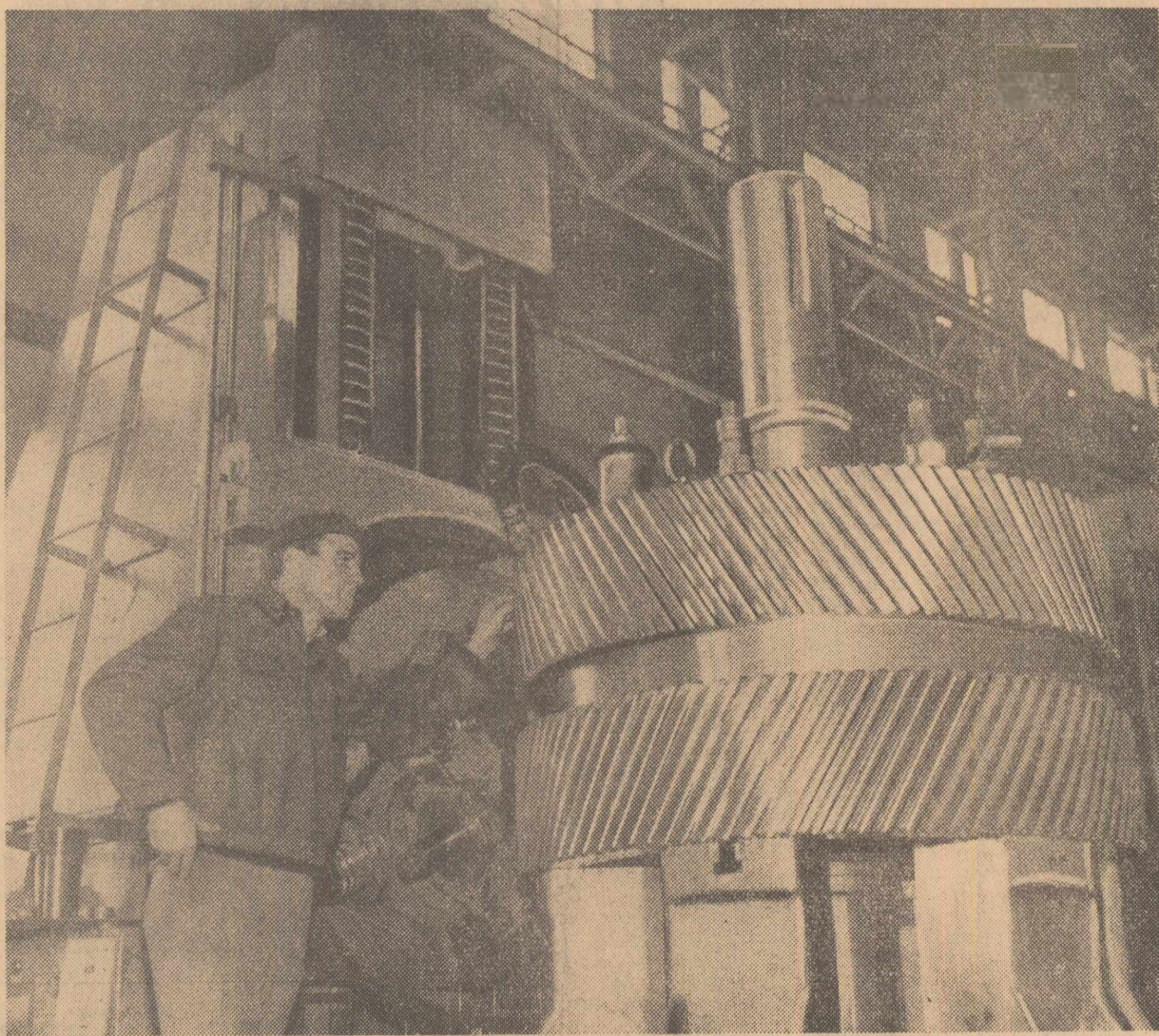
Printre evidențiatii secției construcții mecanice de la Uzina de utilaj greu „Progresul” din Brăila este și frezorul Dumitru Mihai. Cliseul de mai sus îl înfățișează lucrind la frezarea coroanei dințate pentru reductoarele morilor de ciment
