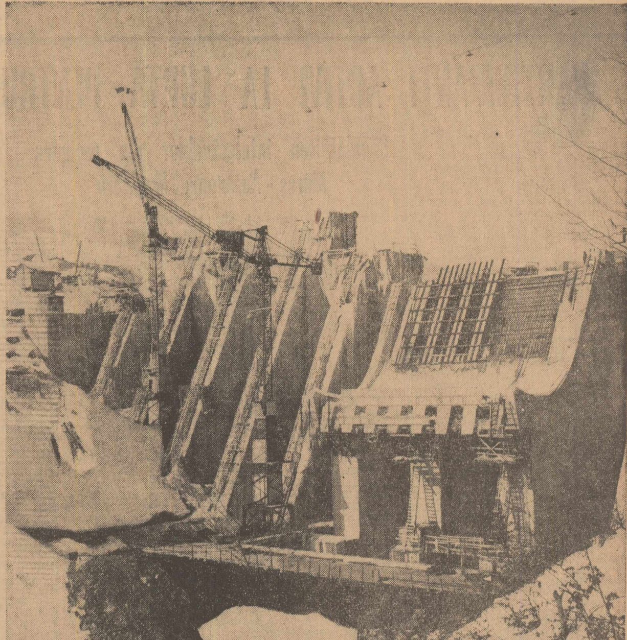
La Firlza — Bala Mare se construiește un mare baraj. Clișeul nostru vă prezintă un aspect de pe acest șantier. Foto: AGERPRES
