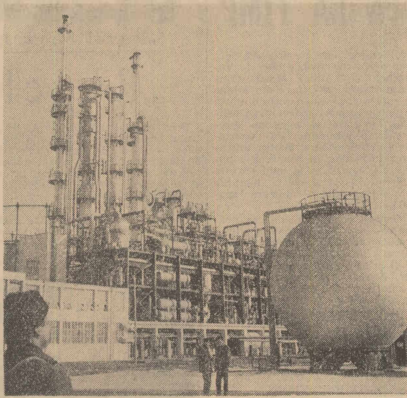
Aspect exterior al instalației de purificare a acetilenei din cadrul fabricii de policlorură de vinil. Foto: AGERPRES
