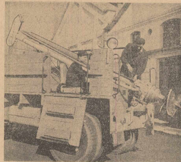
La întreprinderea Energo - reparații din Capitală se fabrică printre altele produse și mașini de săpat gropi și plantat stîlpi, mașini utilizate la montajul liniilor electrice aeriene de 6 Kv și 15 Kv. În elisau: una din aceste mașini de săpat gropi și plantat stîlpi. Foto: AGERPRES
