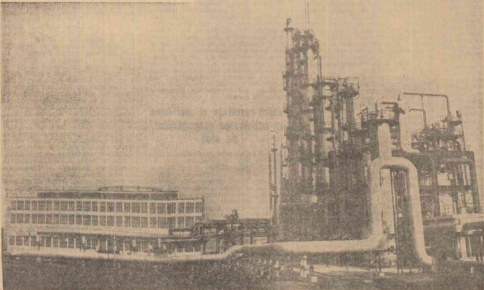
Instalația de purificare a acetilenei din cadrul fabricii de policlorură de vinil, recent intrată în funcțiune
