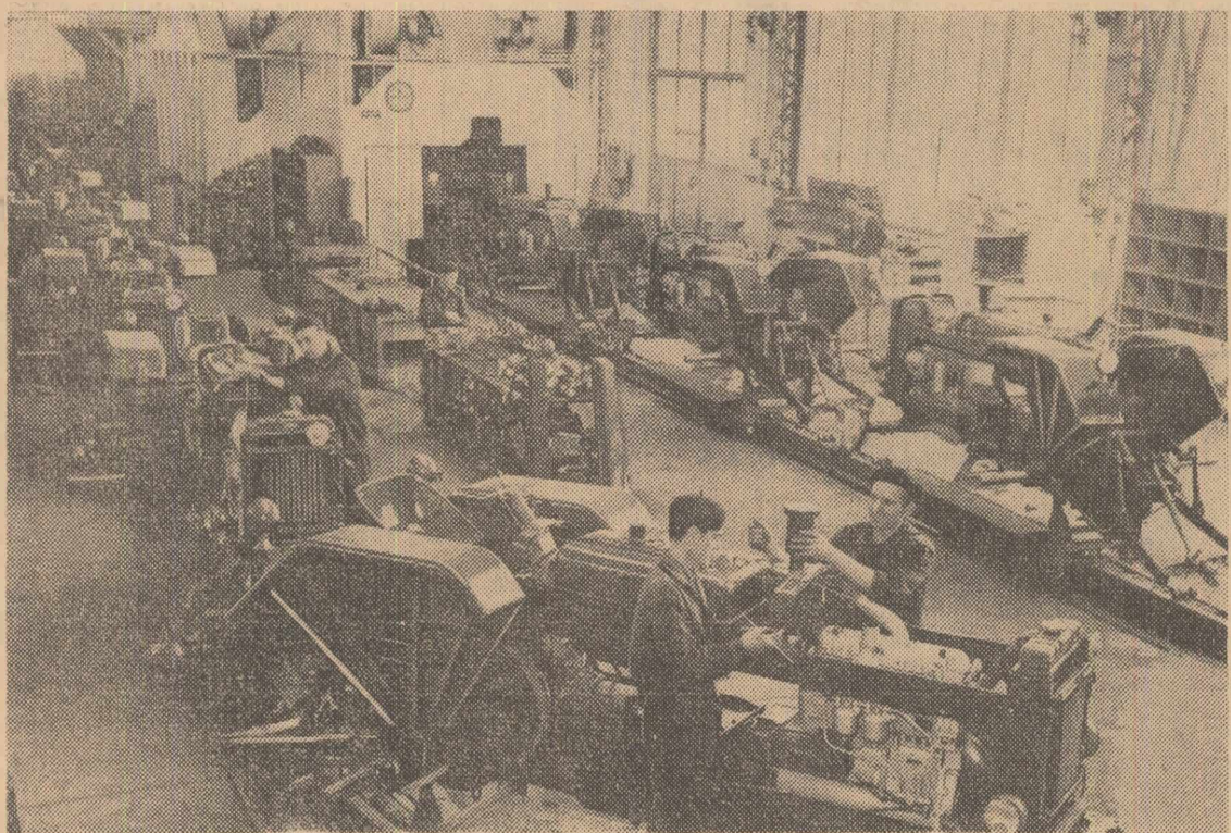
Pe banda de montaj final a tractoarelor
