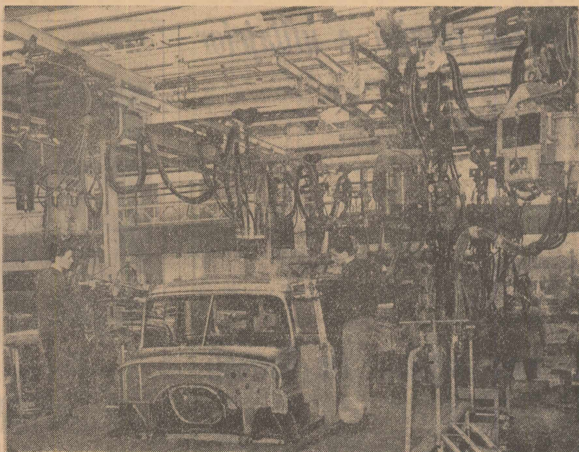
În secția capota a uzinei de autocamioane „Steagul roșu” din Brașov funcționează instalația de sudură automată prin puncte, care asigură o calitate superioară a sudurii precum și o mare productivitate a muncii. În cișeu: Tinerii Steli au Voca și Iosif Tița lucrînd la sudura prin puncte a unei cabine a autocamionului.
