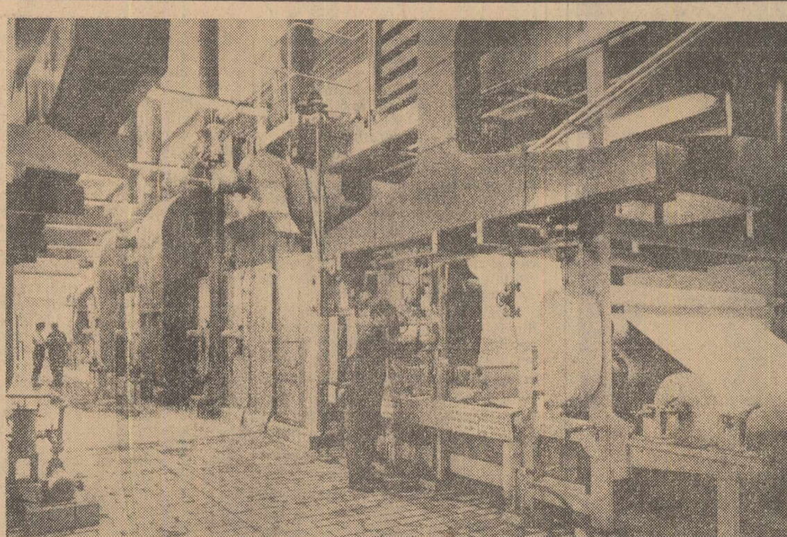
Mașina de impregnare a hîrtiei decorative de la fabrica de înnoibilare a plăcilor fibrolemnoase de la Pipera.
