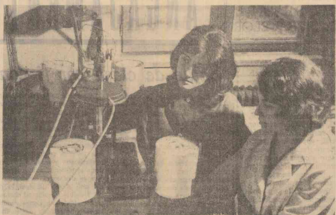
Centrul de cercetări metalurgice al Academiei R.P.R. În laboratorul de tratamente termice ing. Anca Gușu și laboranta Marilena Ionescu lucrînd la o experiență pentru stabilirea cineticii transformărilor izoterme ale oțelului
