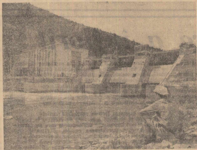
Noile hidrocentrale de pe Bistrița: Roznov II și Pingărați, sînt înzestrate cu turbine romînești, de 7.500 și 11.000 kW, în componența cărora intră piese mari de înaltă tehnicitate ca, de exemplu, carcasa generatorului, camera turbinei, aparatul director, rotorul Kaplan cu palete mobile, sistemul de automatizare etc. Ele sînt dotate cu un sistem de reglaj automatizat de un înalt nivel tehnic. Aceste hidroagregate sînt proiectate și realizate în întregime de metalurgistii uzinelor constructoare de mașini din Reșița. În alîșu: Barajul de la hidrocentrala Pingărați. Foto: AGERPRES
