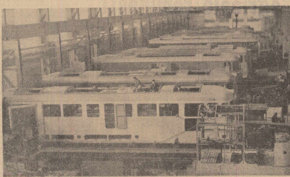
Hala de montaj a locomotivelor diesel-electrice de la uzinele „Electroputere”-Craiova
