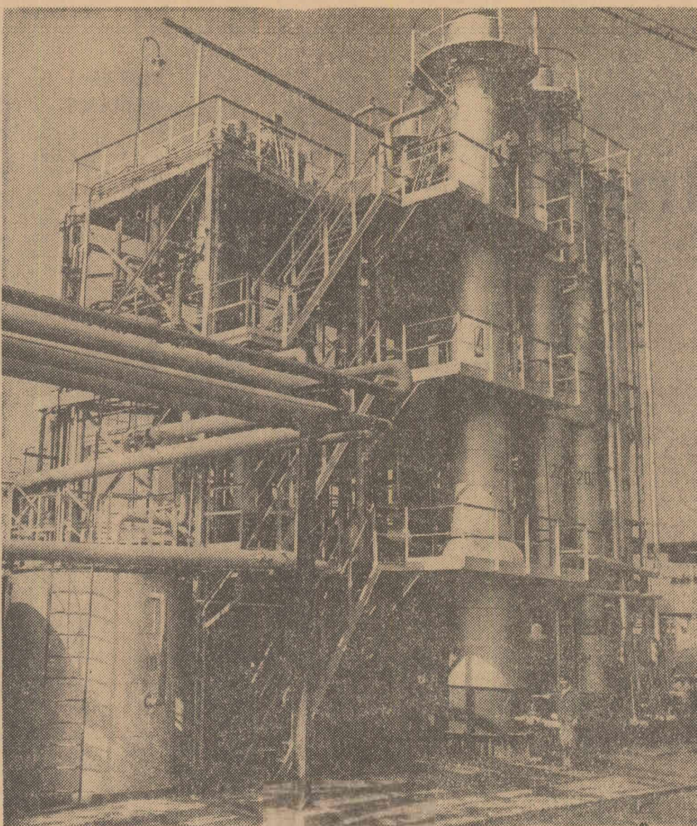
La Uzina de detergenți — Ploiești, a intrat anul acesta în funcțiune o nouă instalație de sulfonare continuă. Astfel, capacitatea de producție a detergenților de tip „Alba” a crescut. În clișeu: Aspect parțial al instalațiilor uzinei de detergenți din Ploiești
