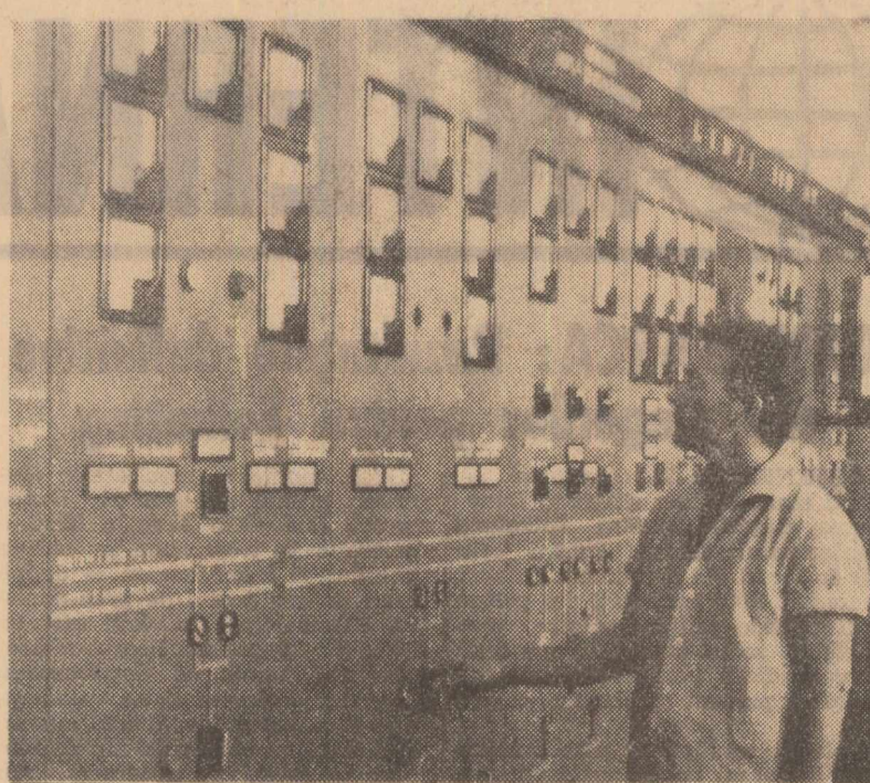
Stația de 110/35 KV — Focșani este o stație de interconexiune și transformare care face legătura dintre Muntenia, Moldova și Dobrogea, asigurînd în acest fel schimbul de energie electrică dintre aceste regiuni. În clișeu: În camera de comandă a stației Focșani
