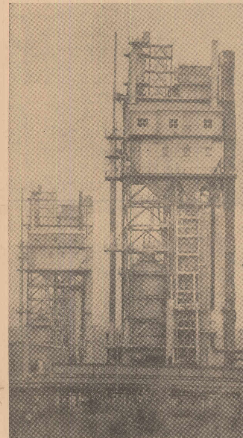
Vederea celor două instalații de oracare catalitică a rafinării Oncoil Foto: NICU VASILE
