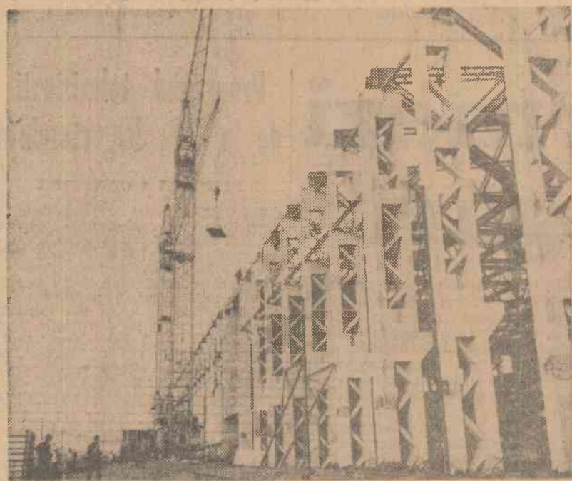
Vedere parțială a unei dintre cele două hale de electroliză (fiecare avînd o lungime de 540 m) de la Uzina de aluminiu Slatina.
