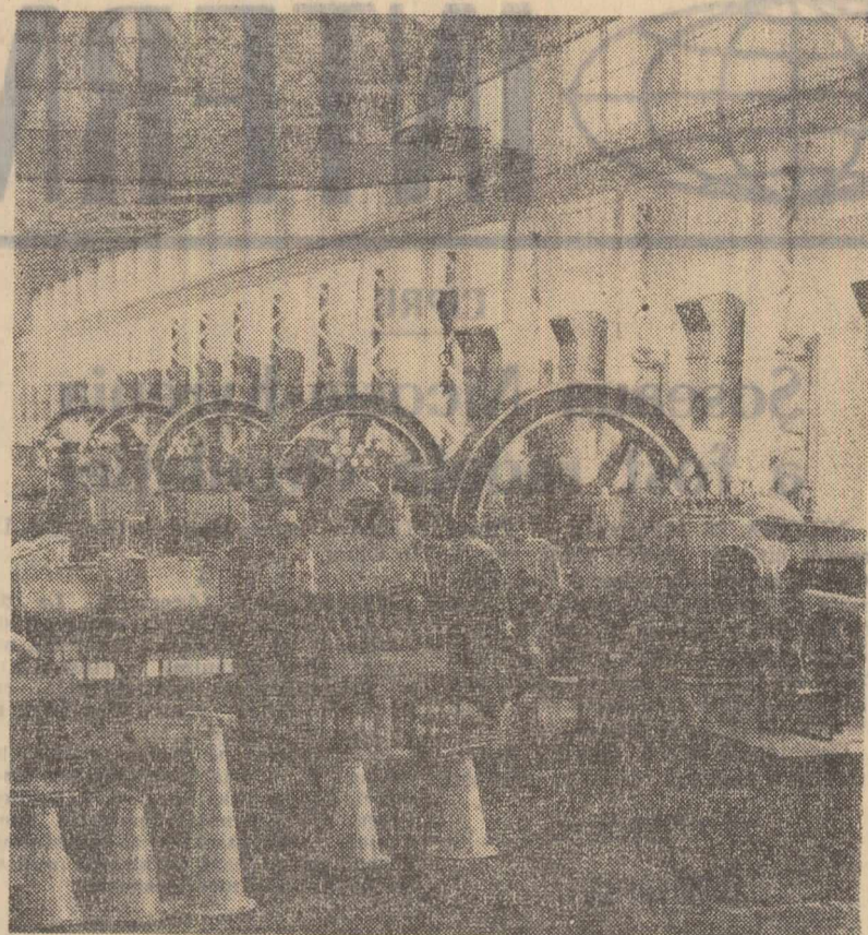
La Combinatul Chimic de la Făgăraș. Aspect din hala de compresoare Foto: N. DUMITRU
