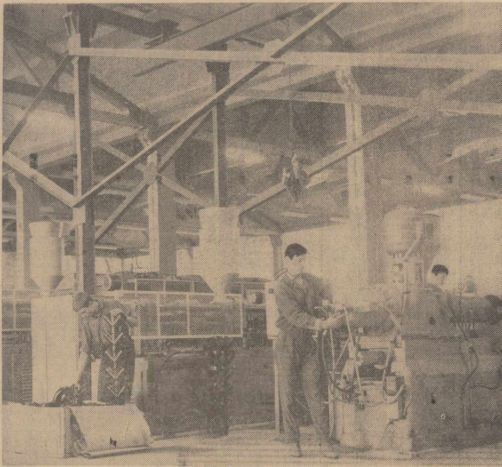
La fabrica de mase plastice din Iași a intrat recent în funcție atelierul de injecție, unde se obțin fitinguri de toate tipurile. Atelierul este dotat cu mașini dintre cele mai moderne, lucrîndu-se în ciclu complet automat. În clișeu: un aspect din acest atelier
