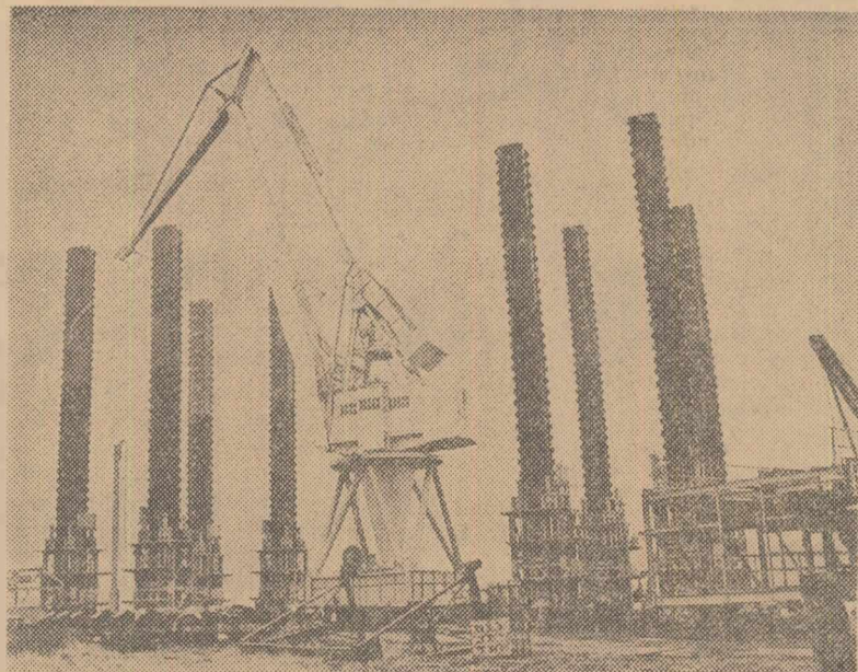
La Schiedam, lângă Rotterdam, în Olanda, a fost construită, de curînd, cea de a doua macara de oțel plutitoare, care va fi utilizată în lucrările de extindere a portului IJmuiden. În fotografie: Macaraua de oțel plutitoare.
