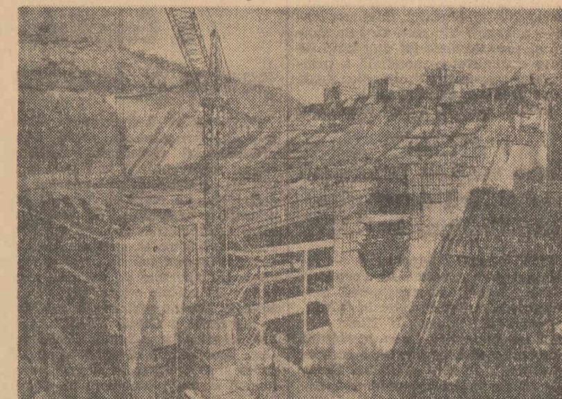
În regiunea munților Rodope, pe riul Arda (R. P. Bulgaria) se ridică barajul „Ivailovgrad”. Iată un aspect de pe șantierul de construcție al barajului.
