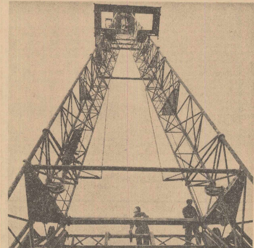
Instalație de foraj 3 DH
