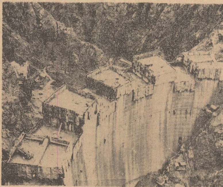
Aspect de la barajul hidrocentralii „16 Februarie” de pe Argeș Foto : P. COZIA
