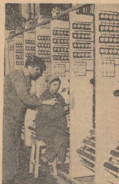
Întreprinderea de construcții metalice și prefabricate nr. 7 din București, produce, printre altele, echipament pentru uzine, stații electrice și linii de înaltă tensiune precum și panouri pentru camere de comandă. În cliseu: Se finalizează panouri destinate unei camere de comandă de 10 KV.
