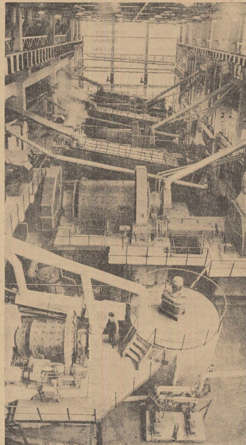
Uzina de alumina Oradea: vedere din secția de măcinare a bauxitei Foto: NICU VASILE
