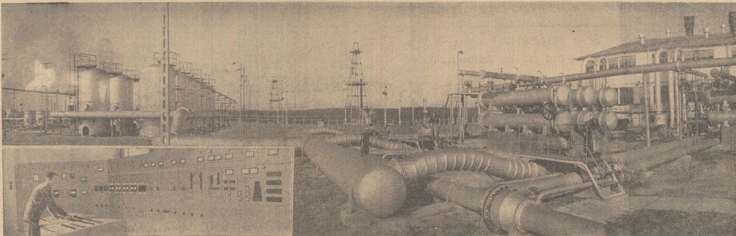
O parte a instalației de desbenzinare a întreprinderii de extracție Țicleni. (În stînga: operatorul Vasile Calotă la pupitrul de comandă)
