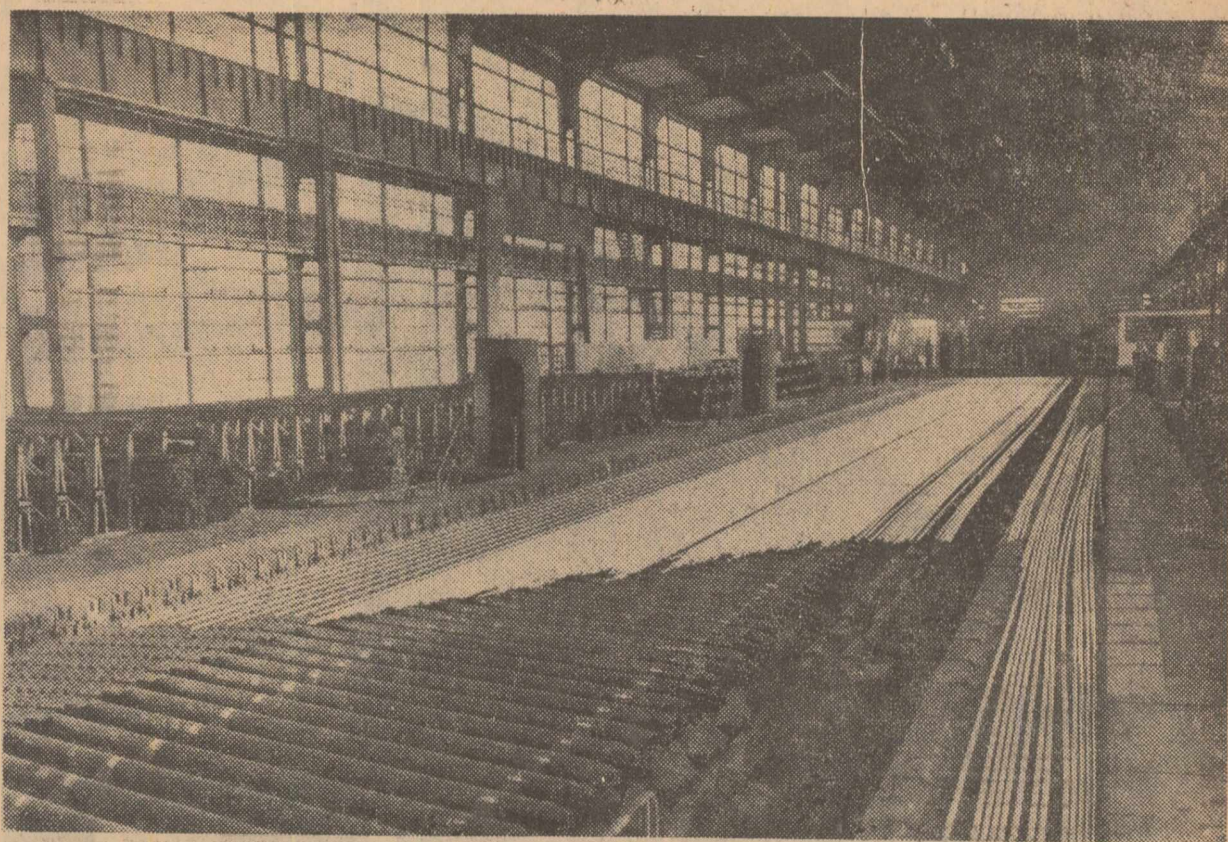
La Combinatul siderurgic din Hunedoara, în lunca Pestișului, se întind pe o mare suprafață halele noulor laminatoare care sînt dotate cu instalații și utilaje moderne de mare productivitate. Aici oțelul este transformat în peste 300 de tipuri de laminare și profile, începînd de la blumuri și prefabricate de oțel, pînă la firele de fier-beton. În clișeu: O vedere de la patul de răcire al laminului de profile fine
