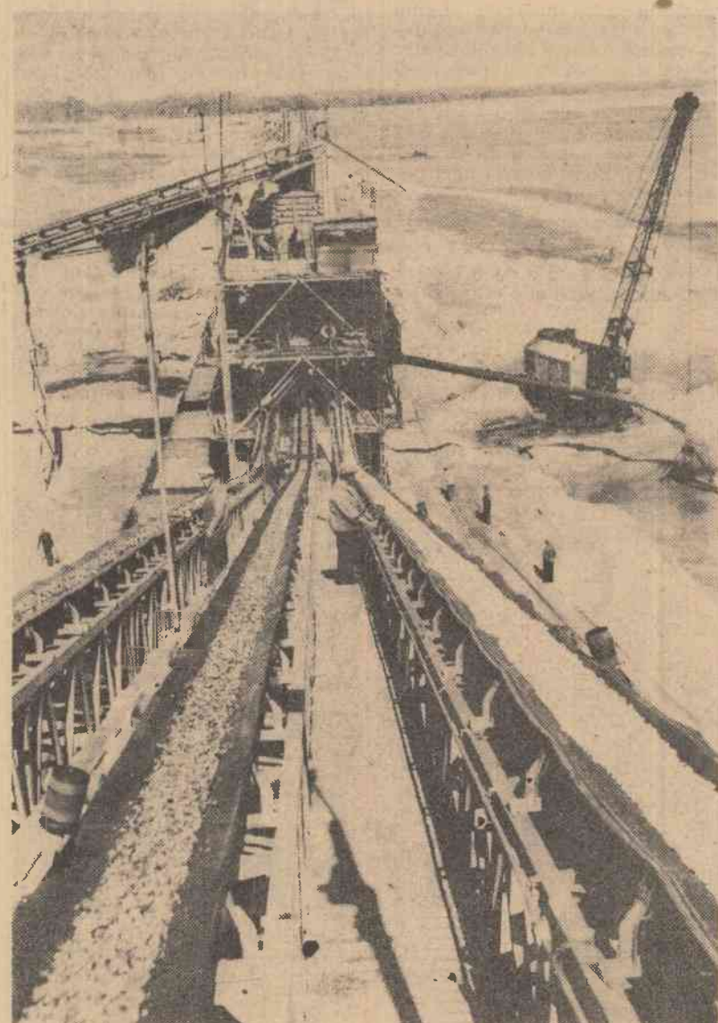
Balastiera Ionești-Găești, așezată pe malul Argeșului, este una dintre cele mai mari și moderne din țară. De aici pleacă zilnic spre marile șantieri ale țării din diferite regiuni, peste 3 500 de tone de produse balastiere sortate. Clișeu nostru înfățișează benziile triple de transport a materialului sortat
