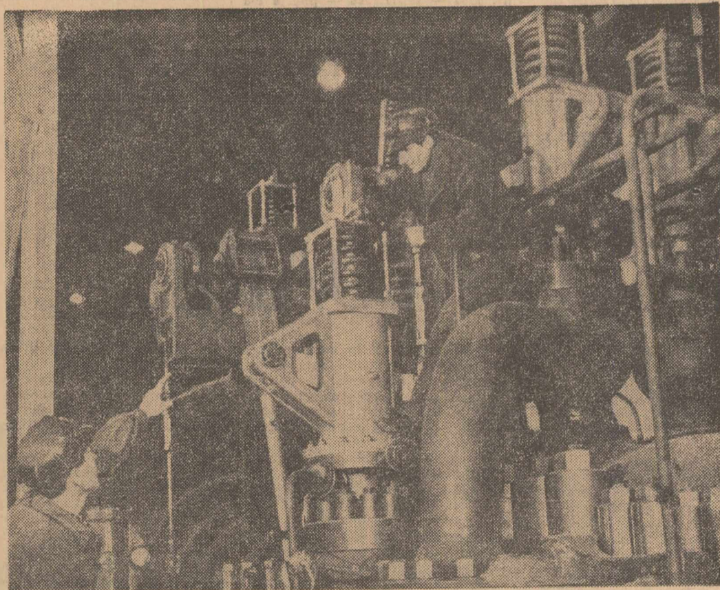
La termocentrala Luduș-Iernut se desfășoară din plin lucrările de montaj ale celui mai mare obiectiv de pe acest șantier. Este vorba de grupul turbogenerator nr. 5 de 200 megawați care se află în preajma probelor mecanice. În clișeu: Șeful de brigadă montor Dumitru Hlastru dînd indicații în timpul primelor probe la acest turbogenerator.
