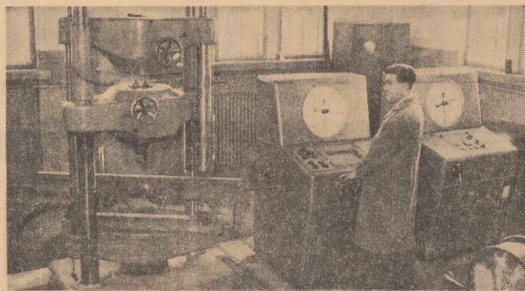
Una din preocupările colectivului Institutului de cercetări C.F.R.-București este și comportarea șinelor sudate. În clișeu: Ing. Victor Ghi meș verifică rezistența la rupere a unei șine sudată prin metoda aluminotermică
