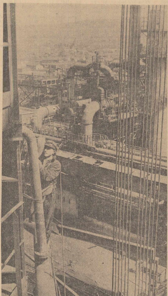
Constructorii și montorii celui mai tânăr agregat siderurgic al Hunedoarei — cel de-al doilea furnal de 1.000 mc. — în timp ce de-a 45-a aniversare a partidului cu înălțarea de seamă. La o serie de lucrări el au anunțat astfel că sint în avans cu stadiul executării. În clădire: Tinarul sudor Cornel Boca lucrând la mare înălțime la instalația de răcire a marelui furnal
