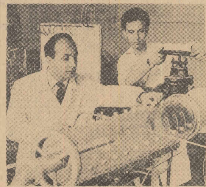
Doi imagini din laboratorul pentru studierea arderii combustibililor gazei, din cadrul Institutului de energetică al Academiei Republicii Socialiste România. Se cercetează caracteristicile de bază ale flăcărilor difuzive: lungime, stabilitate, radiație...
