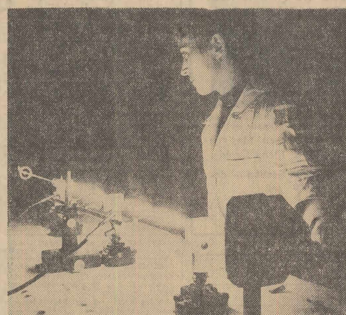
Întă — în funcțiune — un dispozitiv laser cu gaze realizat la Institutul de fizică atomică al Academiei. El urmează să intre în dotarea laboratoarelor marilor uzine, a institutelor de cercetări și a catedrelor din învățămîntul superior
