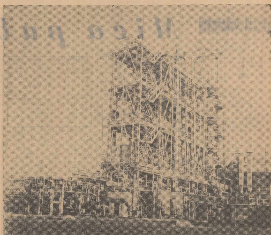
La Combinatul chimic din Craiova au început lu crările de construcție la o serie de noi obiective prevăzute în etapa a doua de dezvoltare; este vorba de fabricile de uree, azotat de amoniu și amoniac.
