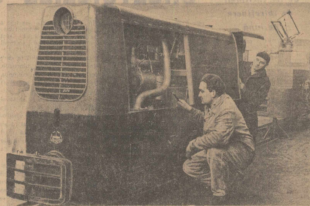
Uzina „Unio” din Satu Mare este specializată în producția de utilaje destinate industriei miniere. Printre produsele modernizate, în ultimul timp, se numără și locomotiva de mină Diesel de 37 C.P. În clădire: Lăcătușii mecanici montori Vasile Bodea și Gh. Holszberger verificînd o locomotivă care va fi expediată la întreprinderea minieră Harghita
