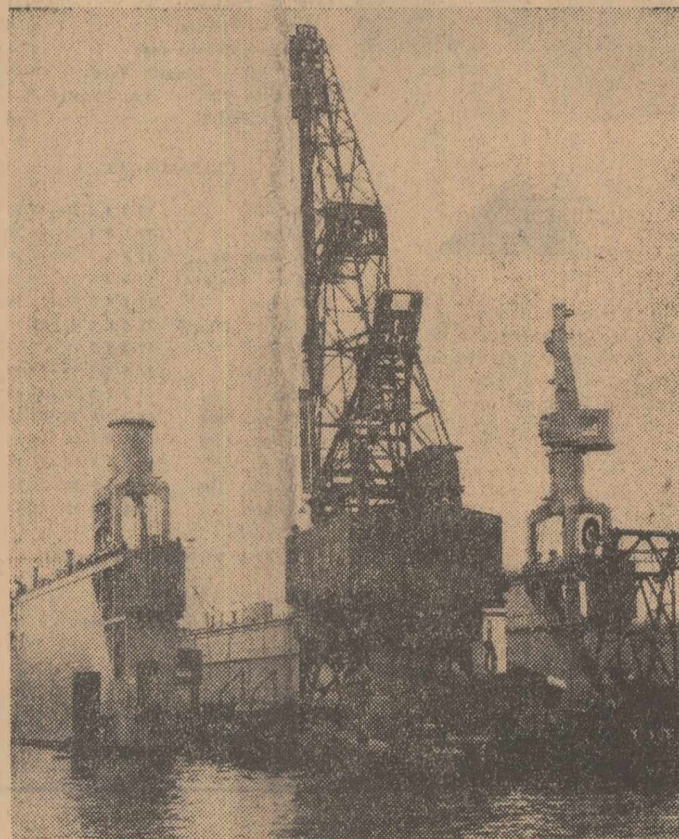
La șantierul naval din Constanța se execută lucrări de montaj și amplasare a unui nou doc plutitor pentru repararea vaselor maritime de diferite tonaje.
