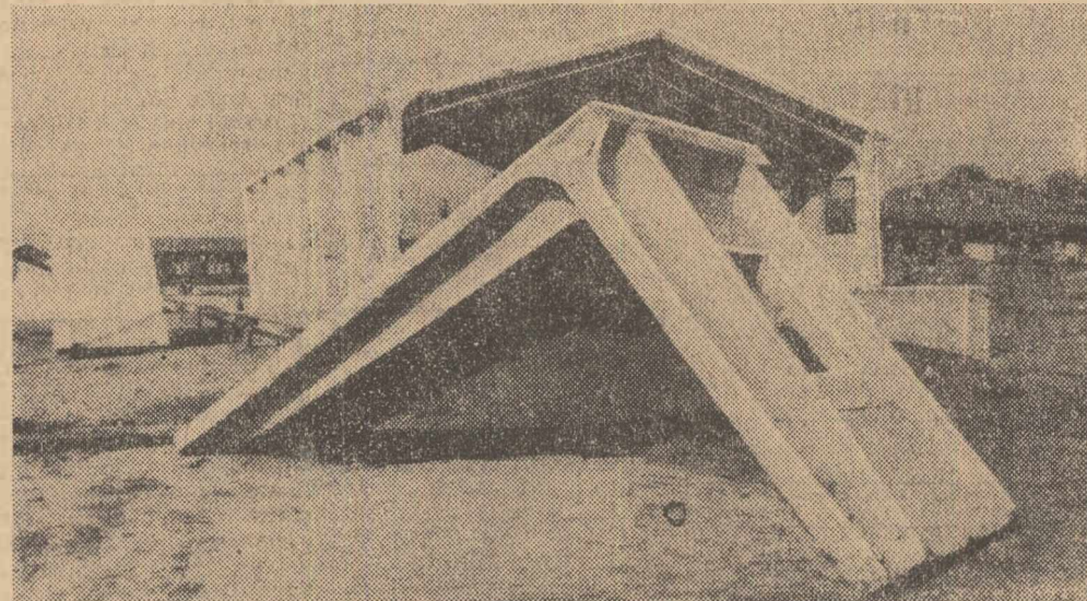
Construcții pentru organizarea de șantier executate la Uzina de fibre sintetice din Iași. În prim plan, un element prefabricat din beton granulat, din care se montează astfel de construcții.
