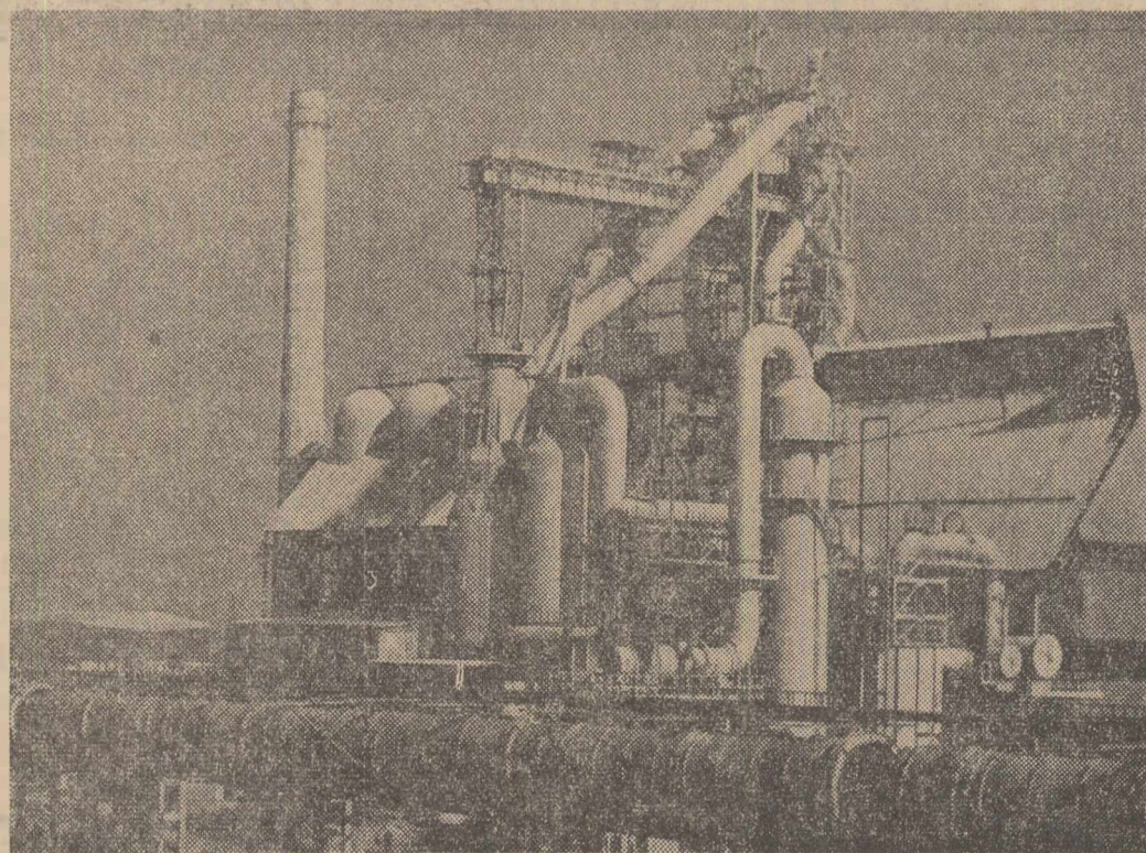
Imaginea de mai sus reprezintă primul furnal de la Combinatul siderurgic „Gh. Gheorghiu-Dej” din Galați, care va intra în funcțiune. Furnalul — cel mai mare agregat siderurgic de acest fel din țară — este proiectat la o capacitate de 1700 mc.
