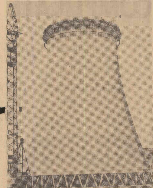
În cadrul lucrărilor la Centrala electrică de termoficare de la Galați a fost executat primul din cele trei turnuri de răcire. Imaginea vă prezintă cofrajul pășitor la cota finală
