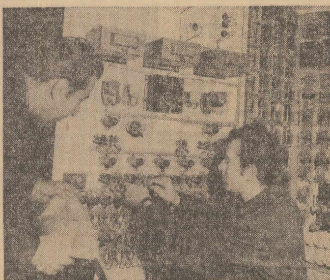
Printre produsele fabricate la Întreprinderea de aparate de măsură și control din Otopeni-București se numără și panourile de automatizare pentru stațiile de irigare din agricultură, care asigură automatizarea completă în sistemele mari de irigare. Panourile sînt echipate cu aparatură de concepție românească. În clipă: ministrul Florin Olaru explică muncitorilor electrician Marinov Gheorghe parcurse funcțională a schemei panoului de automatizare.
